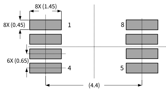
MSOP8
