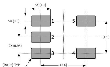
SOT23-5L
