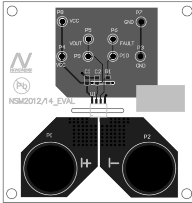
Figure 7.3 NSM2012-Q1 PCB Layout
