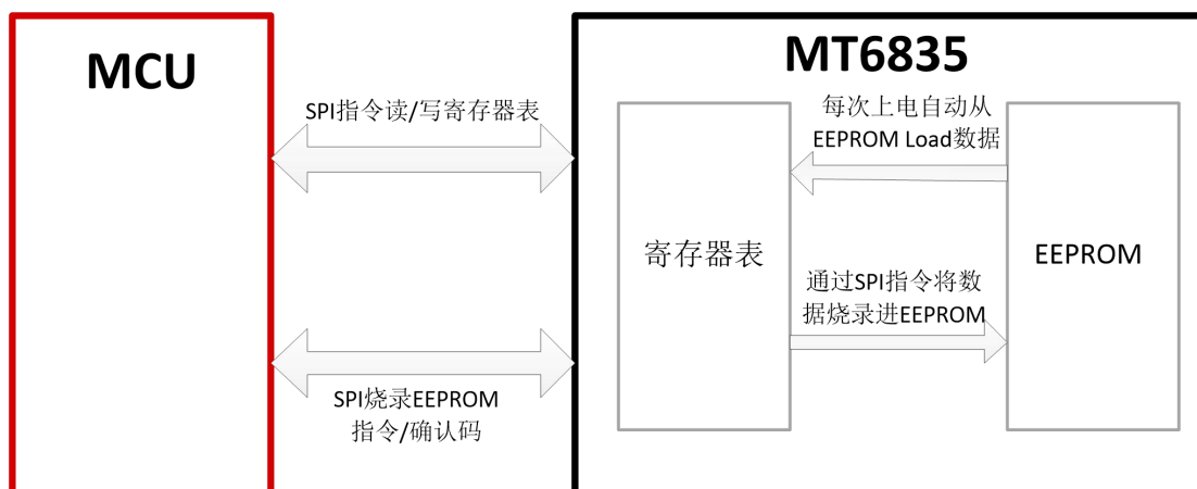
图-22: 寄存器表和EEPROM关系
