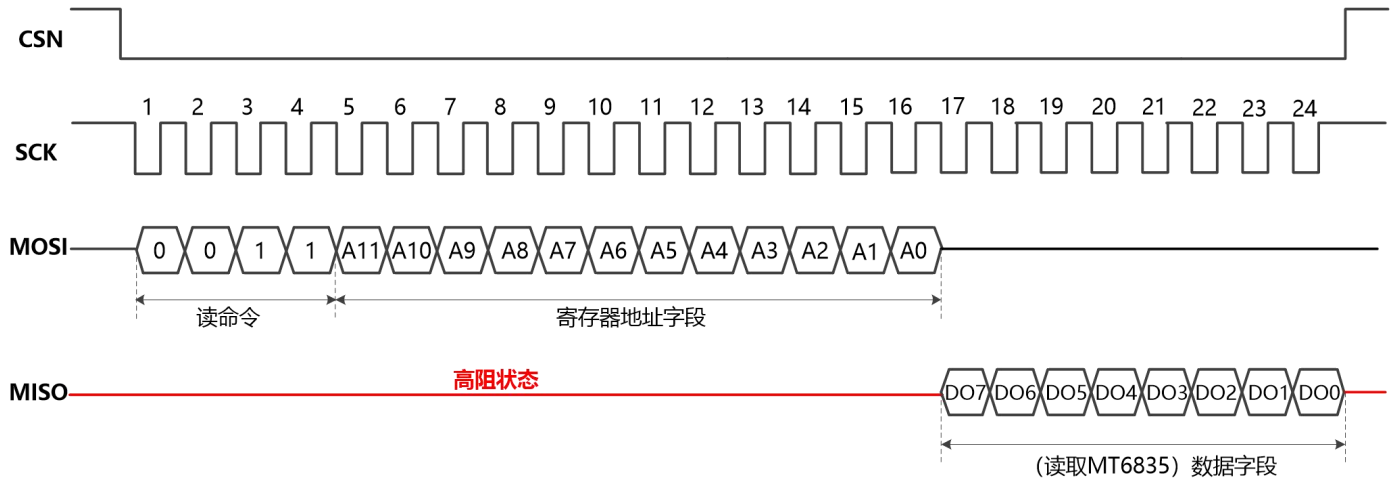
图-19: SPI单字节读寄存器
