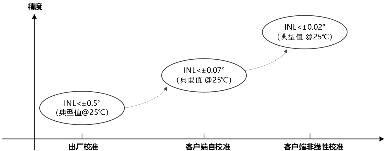
图-27: 三层校准
