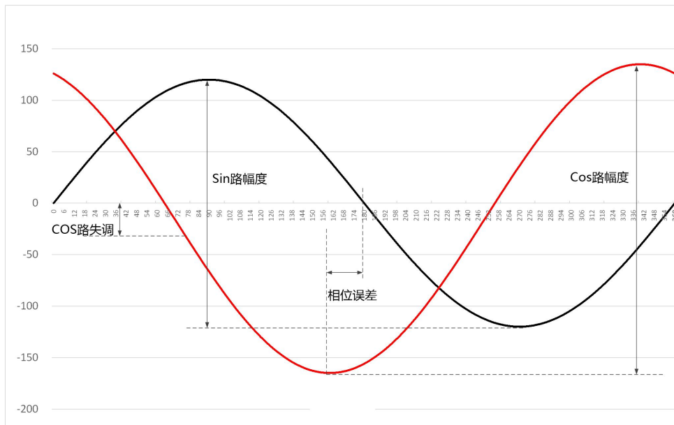
图-28: 失调、幅度误差和相位误差
