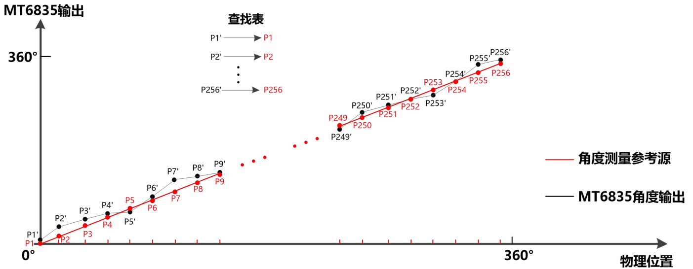
图-29: 客户端非线性校准
