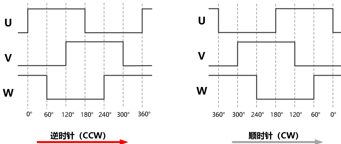
图-14: UVW输出波形
