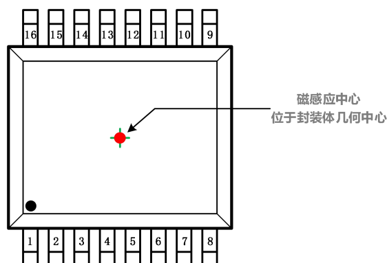
图-1: MT6835 TSSOP-16封装外观图
