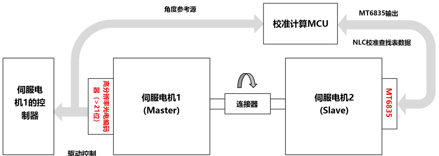
图-30: 一种推荐的客户端非线性校准对拖系统
