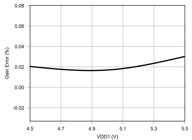
Figure 6.21 EG vs VDD1
