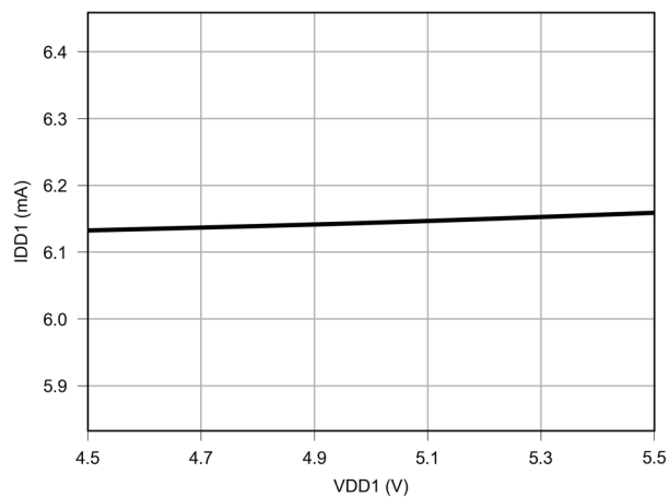
Figure 6.24 IDD1 vs VDD1
