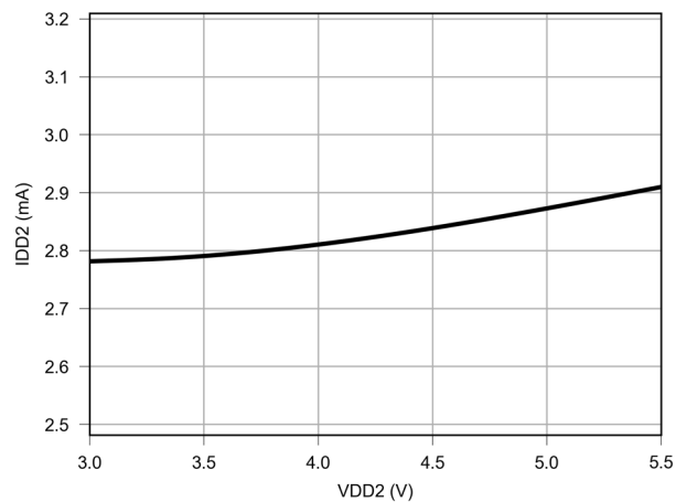
Figure 6.25 IDD2 vs VDD2
