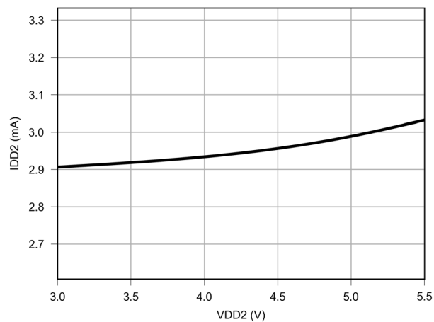
Figure 6.10 IDD2 vs VDD2
