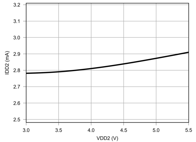
Figure 6.25 IDD2 vs VDD2
