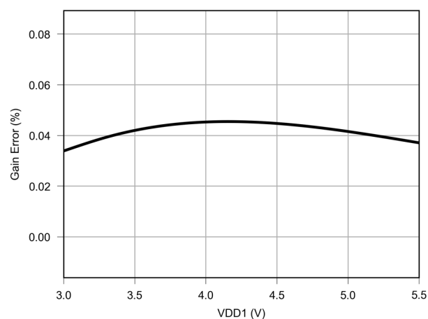
Figure 6.6 EG vs VDD1
