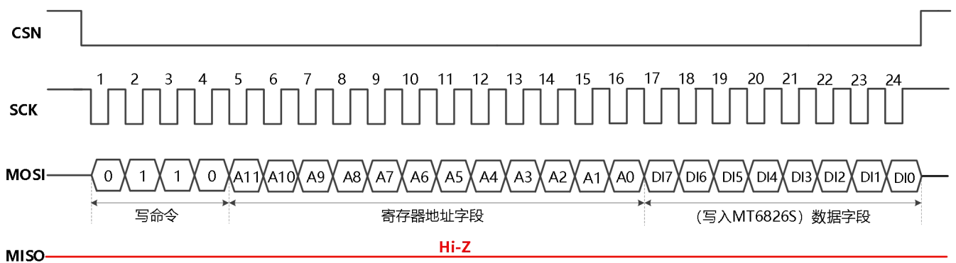
图-21: SPI单字节写寄存器
