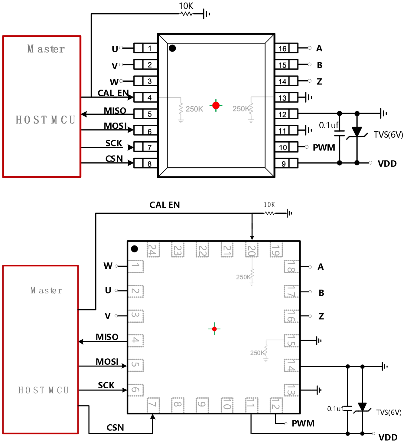
图-7: 参考电路 (客户端做自校准)
