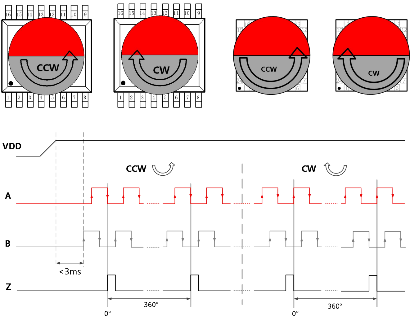
图-8: ABZ输出模式
