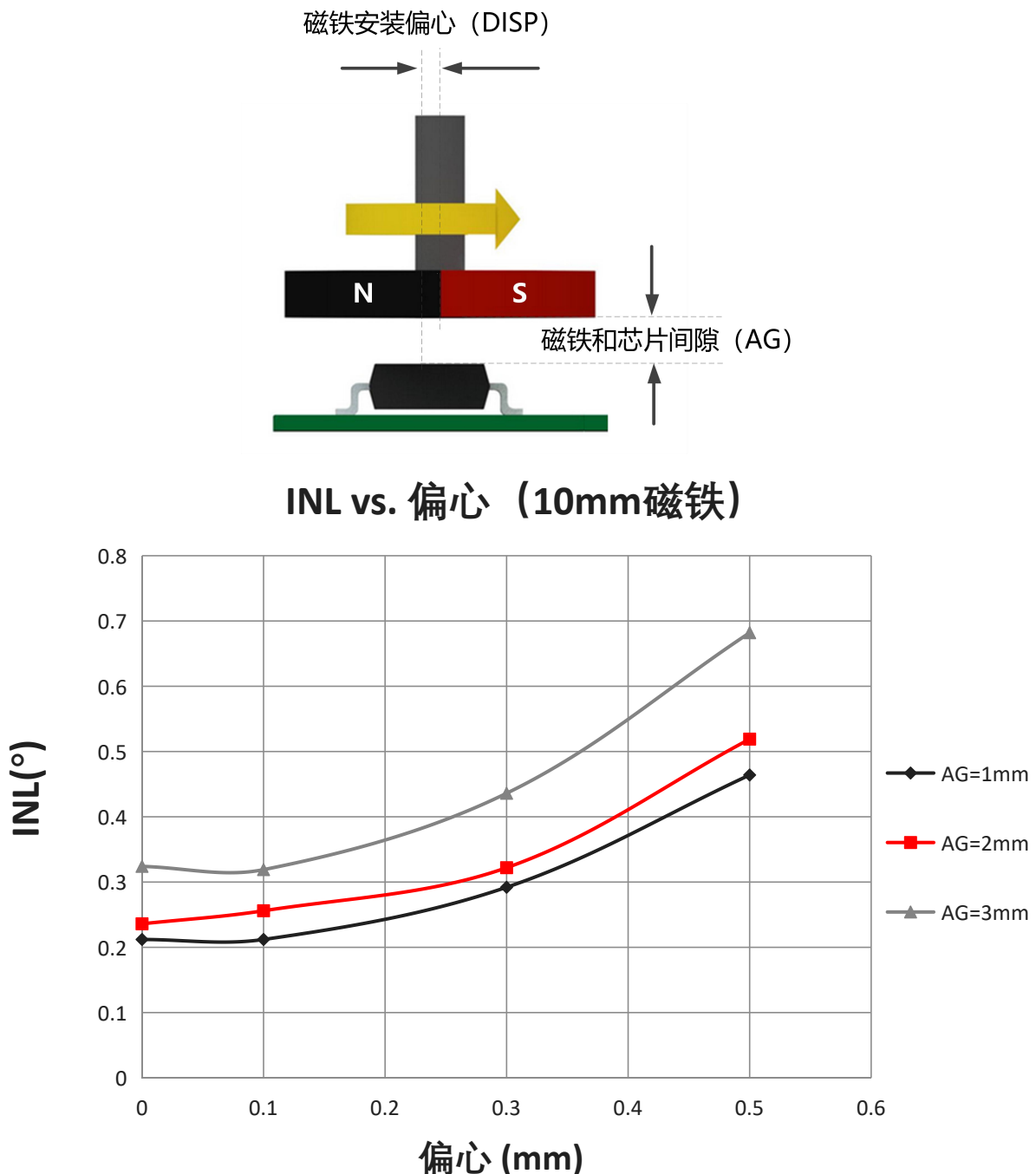
图-30: INL vs. 偏心和间隙变化的表现 (仅做了出厂校准)
