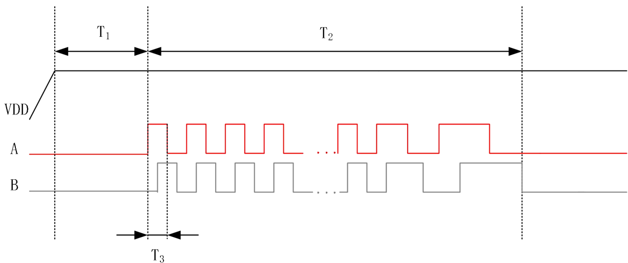
图-27:AB信号上电输出绝对角度示意图
