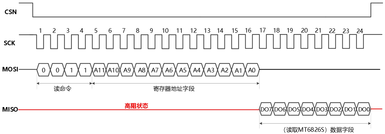
图-20: SPI单字节读寄存器
