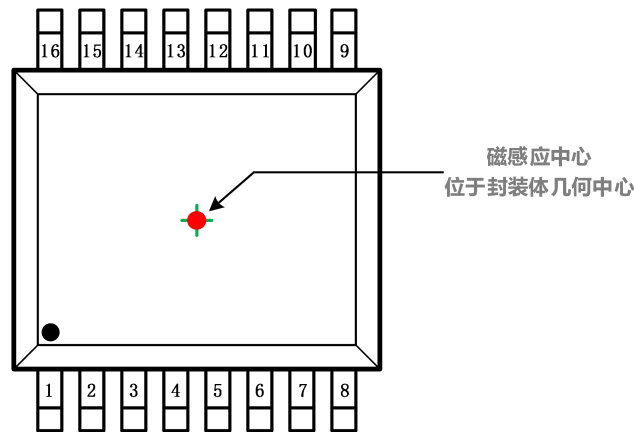
图-1: MT6826S TSSOP-16封装外观图
