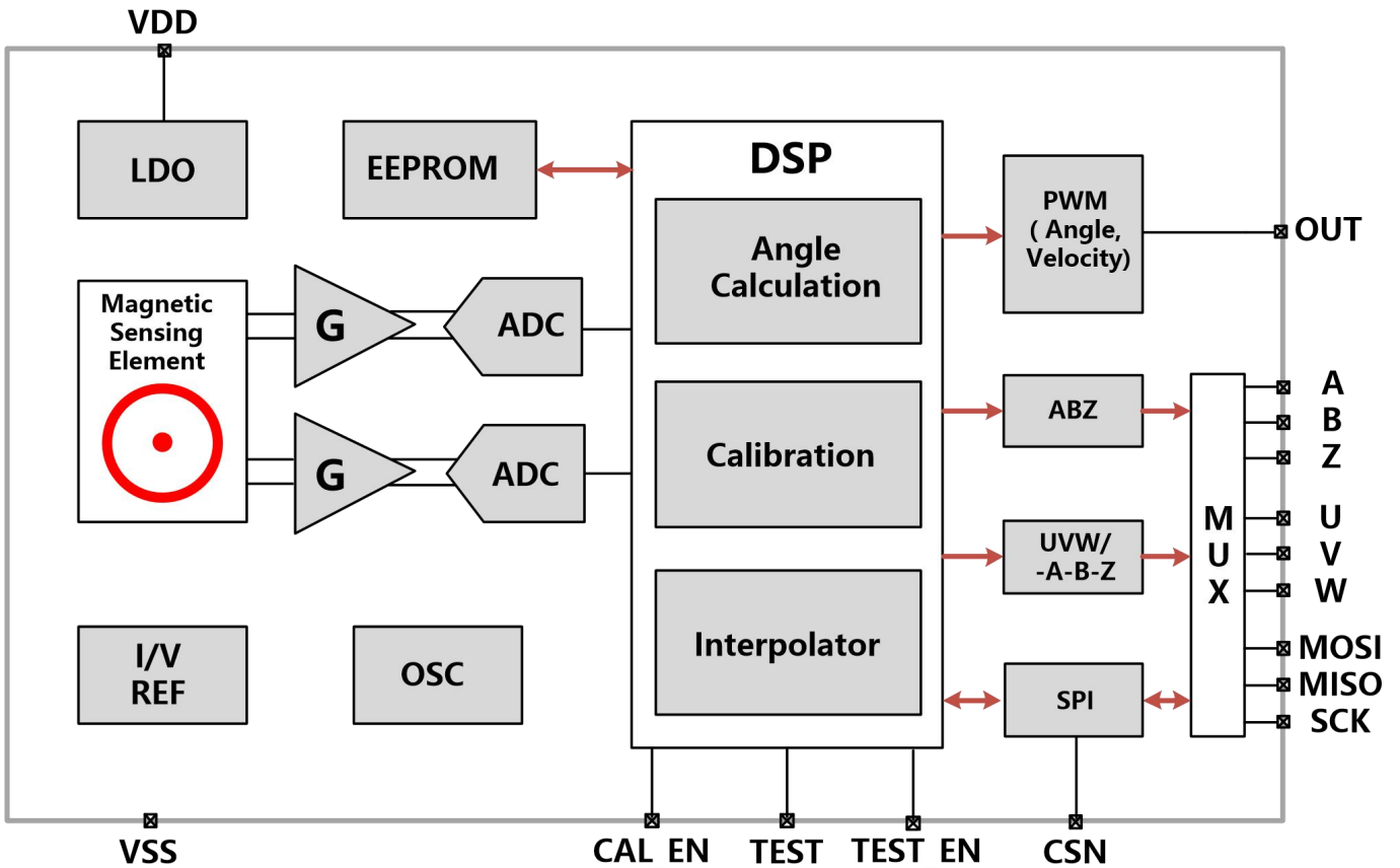
图-3: 芯片功能框图
