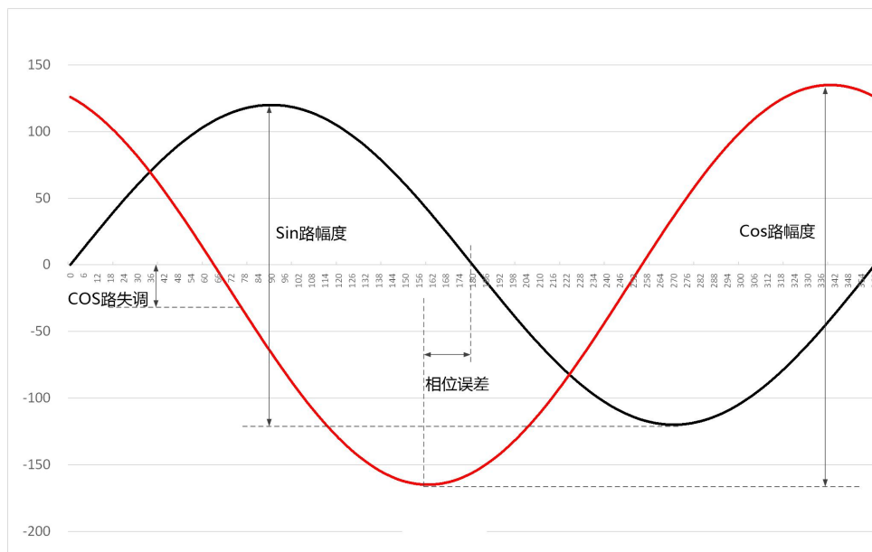
图-29: 失调、幅度误差和相位误差
