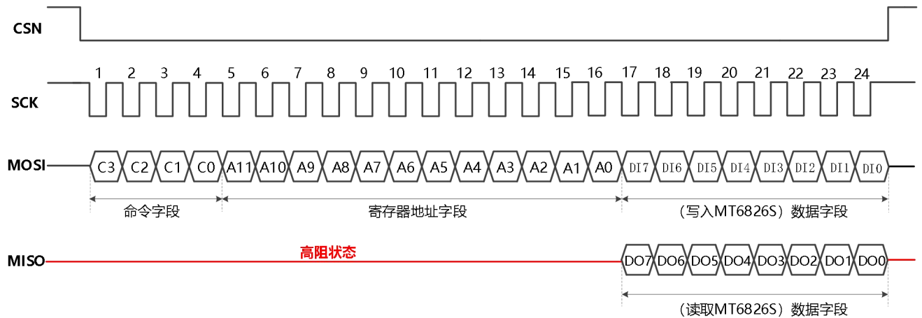
图-19: 4线SPI协议时序
