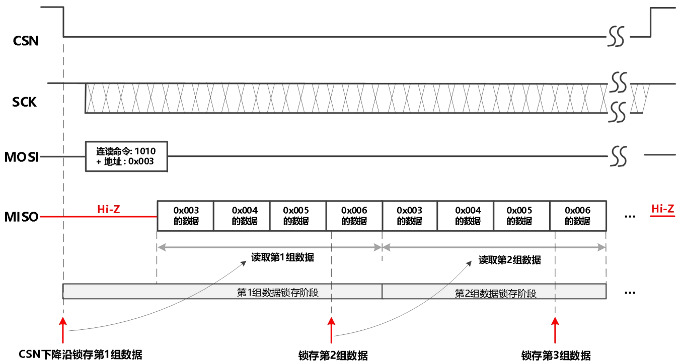
图-25: SPI 连续角度寄存器数据
