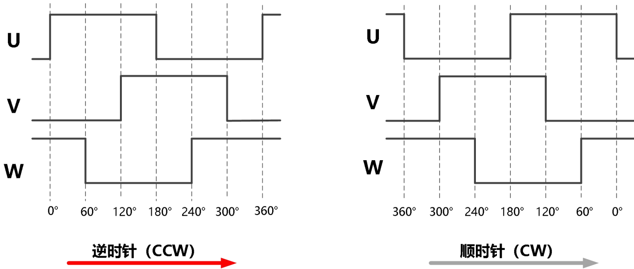
图-15: UVW输出波形
