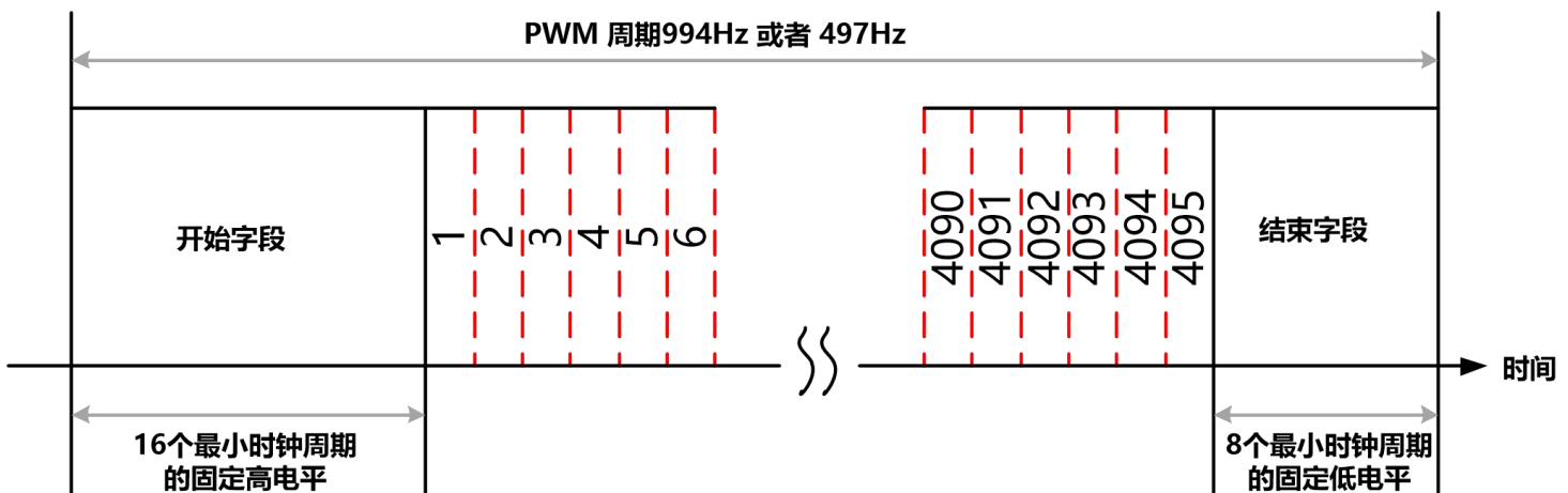
图-16: PWM输出
