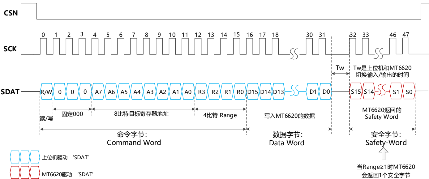
图-15: 3线SPI写操作
