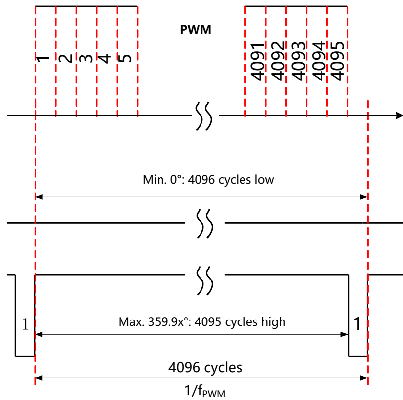
图-12: PWM输出
