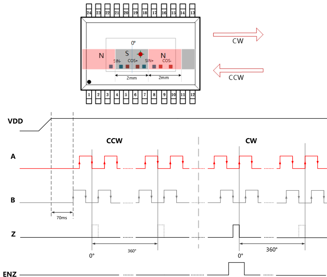
图-6: ABZ输出
