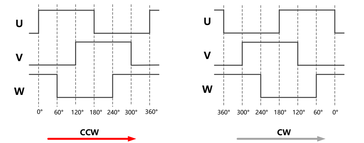
图-11: UVW输出波形
