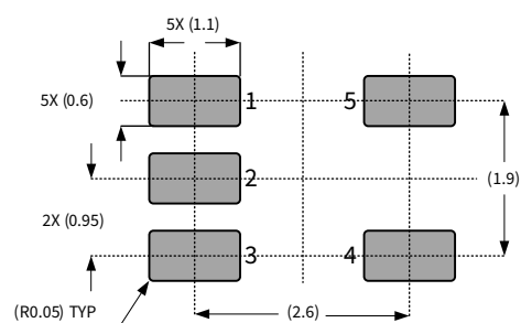
SOT23-5L
